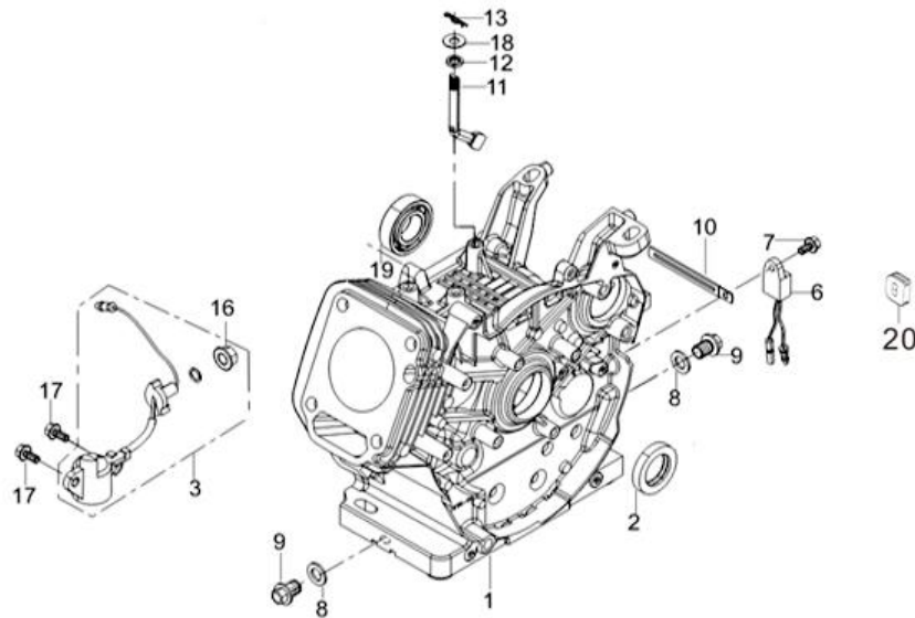
图1：曲轴箱组件(E01)
