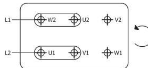
Senso di rotazione antiorario Counterclockwise rotation
