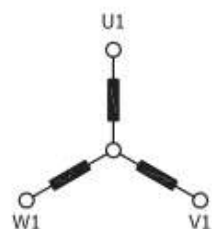
Collegamento Y Y Connection
