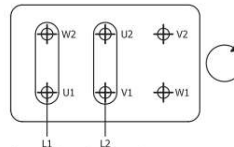
Senso di rotazione orario Clockwise rotation
