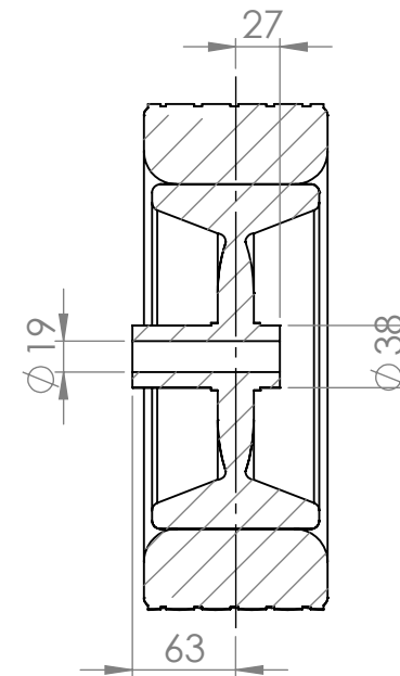
SECTION A-A
