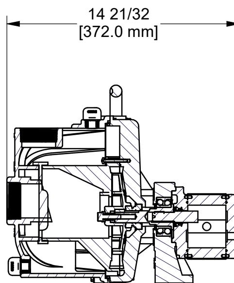
SECTION A-A SCALE: 1/4
